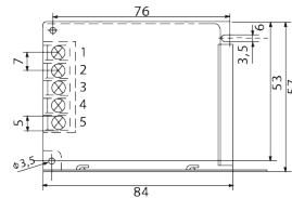
VOEDING 24Vdc - 60W max
