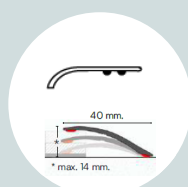
Detail transitieprofiel
