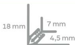
Tweedelig binnenhoekprofiel 2600 mm
