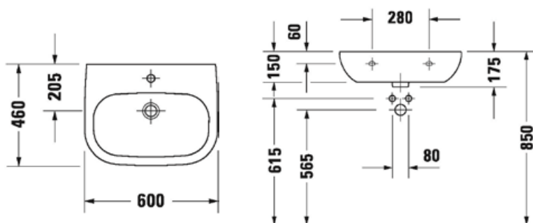
Technische tekening DU23116000002
