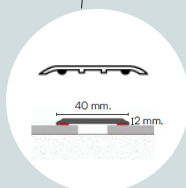
Detail expansieprofiel
