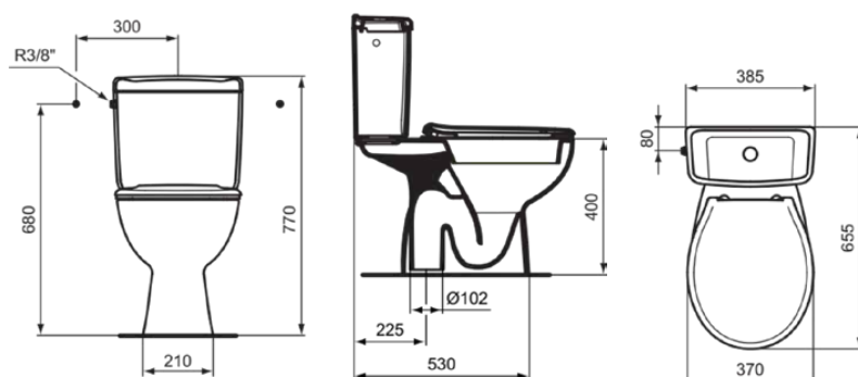
Verticale uitgang
