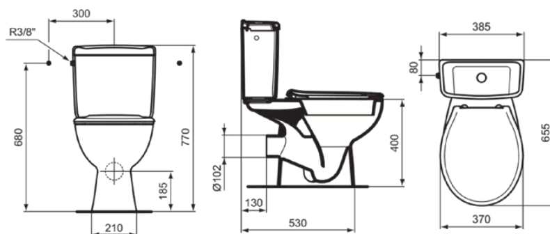
Horizontale uitgang
