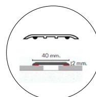
Detail expansieprofiel
