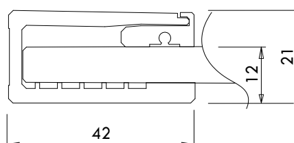
STANDAARDPROFIEL
