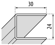
LUNES H H 195 cm GIADA H H 195 cm
