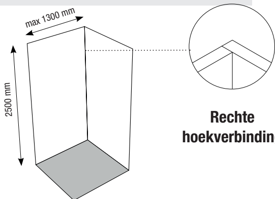
Recht paneel
