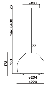
Versie Ø 22 cm
