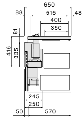
Zijaanzicht
