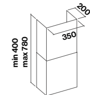
Schacht optioneel
