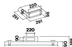
Aansluitstuk (KACL.789)
