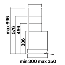
Zijaanzicht met optionele schacht
