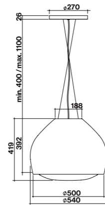
Versie Ø 54 cm*
