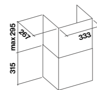
Optioneel schacht
