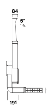
Zijaanzicht, Slim motor achter
