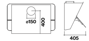
Achteraanzicht
