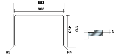
Vlak inbouw Gatmaat
