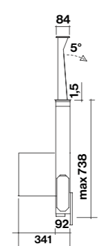
Zijaanzicht, motor aan achterkant
