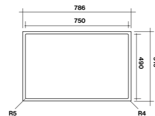
Vlak inbouw afmetingen
