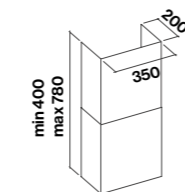
Schacht optioneel
