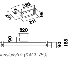
Aansluitstuk (KACL.789)
