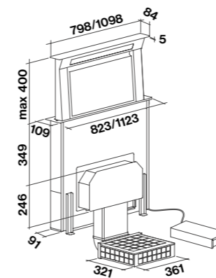
Uitsparing 90 cm: 98 mm x 810 mm 120 cm: 98 mm x 1110 mm
