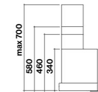
Zijaanzicht met optionele schacht
