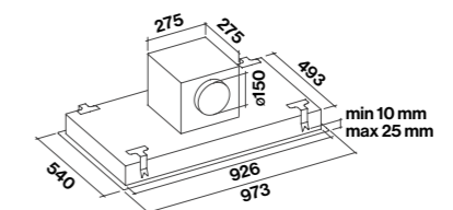
Aansluitstuk (KACL.789)
