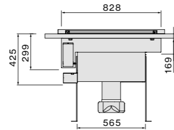
Vooraanzicht
