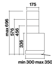
Zijaanzicht met optionele schacht
