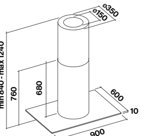
Eiland versie met glas (optioneel)
