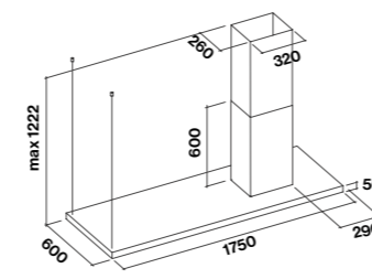
Rechters versie
