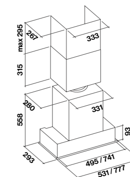
Uitsparing: 50 cm: 506 mm x 262 mm 70 cm: 751 mm x 262 mm
