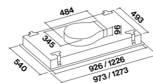
Externe doorvoer motor KACL.798#41F
