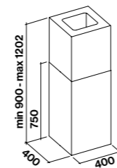
Eiland versie
