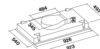
Externe doorvoer motor KACL.798#41F
