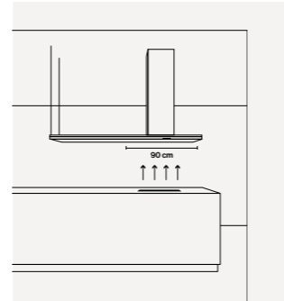
Afzuig oppervlak is 90 cm, rechts onder de schacht
