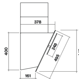
Zijaanzicht
