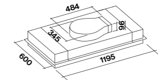
Externe doorvoer motor KACL.798#41F
