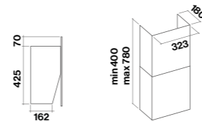
Zijaanzicht
