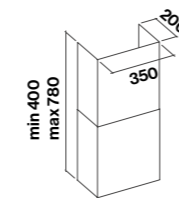
Schacht optioneel
