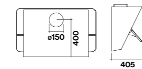
Achteraanzicht
