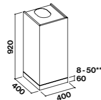
Wand versie
