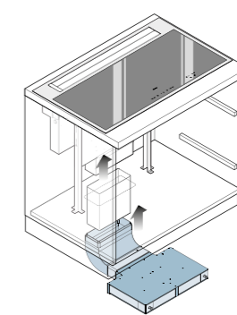
Plint filter h60 (KACL.951)
