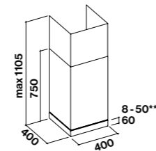
Wand telescopische versie **Aanpasbare opening
