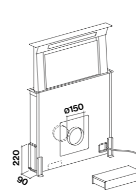
Installatie voorbeelden.
