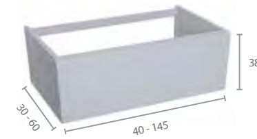
TB4 Geen uitsparing voor sifon Sans découpe pour siphon
