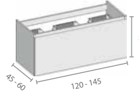
A2B.02 2 uitsparingen voor sifons 2 découpes pour siphons
