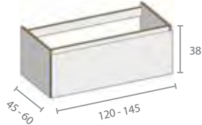
A4.02 2 uitsparingen voor sifons 2 découpes pour siphons
