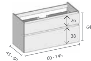
A7.01 1 uitsparing voor sifon 1 découpe pour siphon
