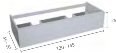
TA1.02 2 uitsparingen voor sifons 2 découpes pour siphons
