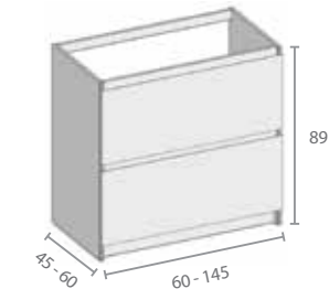
A8.01 1 uitsparing voor sifon 1 découpe pour siphon
