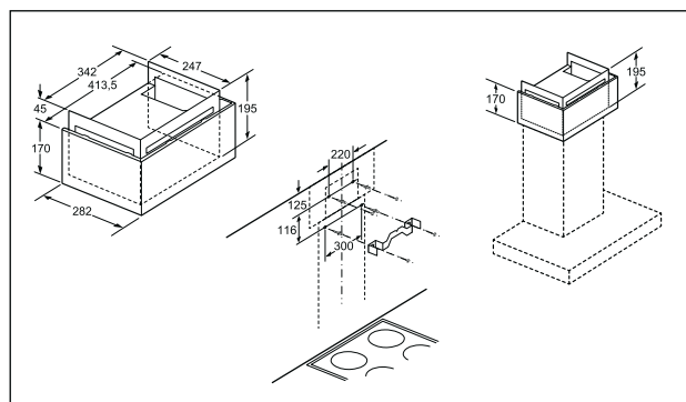
Inbouwschema CleanAir Plus-Set voor wanddampkappen
