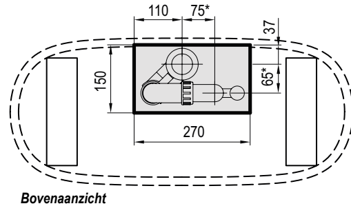
Bovenaanzicht
