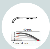
Detail transitieprofiel
