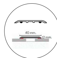
Detail expansieprofiel
