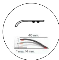
Detail transitieprofiel
