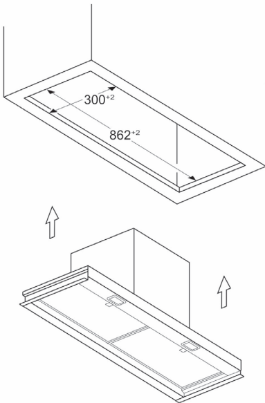
Afmeting in mm Installatievoorbeeld in meubeluitsparing
