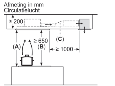
A: Optimale prestaties 700-1500 B: Vanaf bovenkant pannendrager C: Verbindingsstuk (van een rechthoekig kanaal naar een rond kanaal). Wordt niet meegeleverd.
