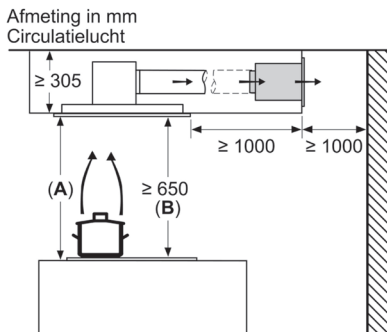
A: Optimale prestaties 700-1500 B: Vanaf bovenkant pannendrager
