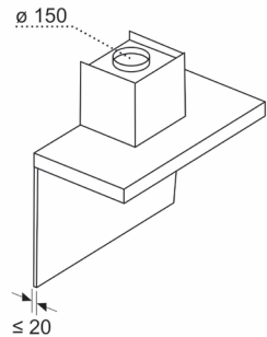
Afmeting in mm Wandpaneeldiepte
