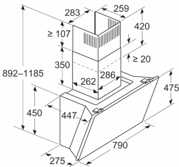
Afmeting in mm Apparaat in luchtcirculatiemodus
