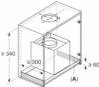
Afmeting in mm Installatievereisten voor vervanging
