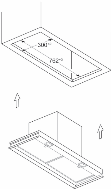
Afmeting in mm Installatievoorbeeld in meubeluitsparing
