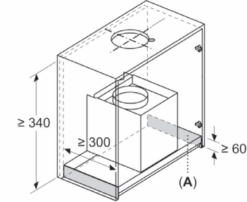
Afmeting in mm Installatievereisten voor vervanging
