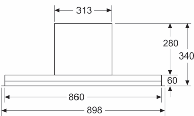
Afmeting in mm Vooraanzicht
