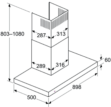
Afmeting in mm Recirculatieperspectief
