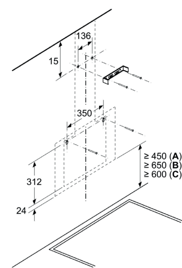
Afmeting in mm Wandinstallatie met luchtkanaal
