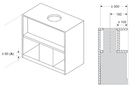
Afmeting in mm Installatievoorbeeld met kruidenrek
