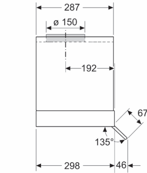
Afmeting in mm Zijaanzicht
