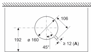
Afmeting in mm Aanzicht van boven
