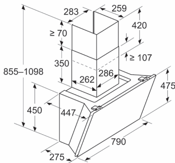
Afmeting in mm Apparaat in luchtafvoermodus
