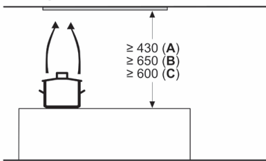
Afmeting in mm
