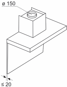
Afmeting in mm Wandpaneeldiepte
