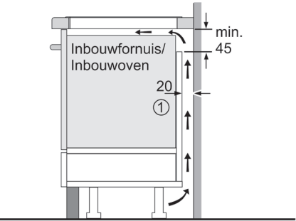
Afmetingen in mm
