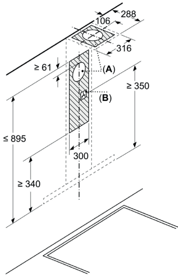
Afmeting in mm
