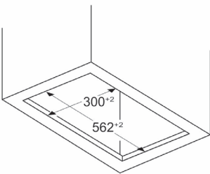
Afmeting in mm Installatievoorbeeld in meubeluitsparing
