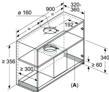
Afmeting in mm Inbouwvoorbeeld
