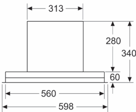
Afmeting in mm Vooraanzicht
