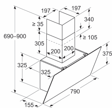
Afmeting in mm Apparaat in luchtafvoermodus
