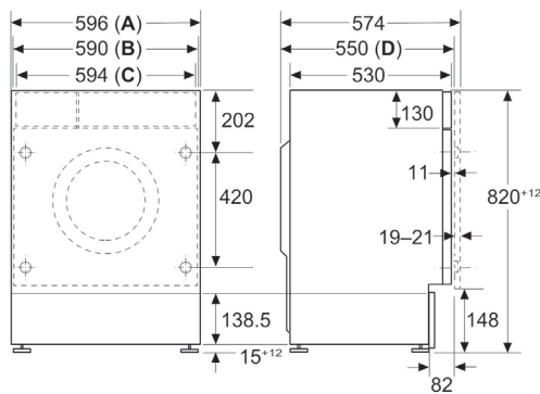
B: Gatdiepte scharnieruitsparing min. 12 mm diep
