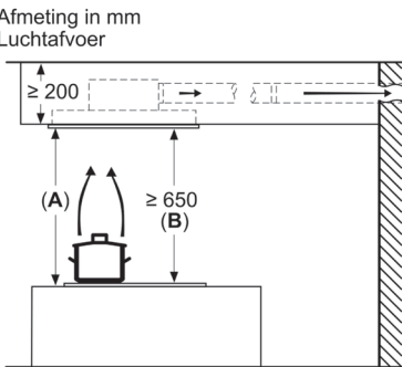
A: Optimale prestaties 700-1500 B: Vanaf bovenkant pannendrager
