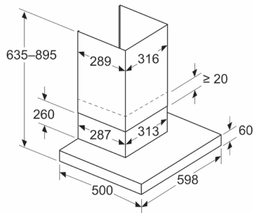
Afmeting in mm Apparaat in luchttafvoermodus
