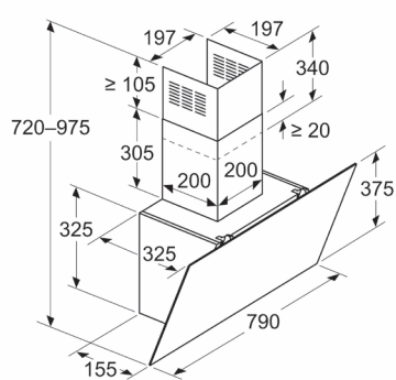
Afmeting in mm Apparaat in luchtcirculatiemodus
