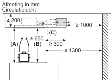
A: Optimale prestaties 700-1500 B: Vanaf bovenkant pannendrager C: Verbindingsstuk (van een rechthoekig kanaal naar een rond kanaal). Wordt niet meegeleverd.
