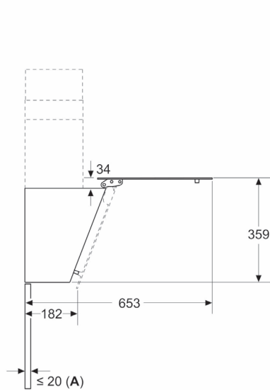
Afmeting in mm
