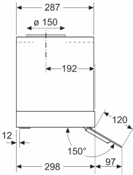
Afmeting in mm Zijaanzicht
