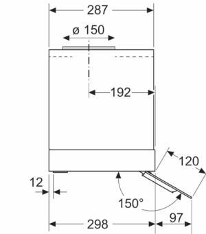
Afmeting in mm Zijaanzicht
