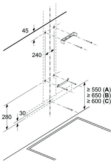
Afmeting in mm Wandinstallatie met luchtkanaal
