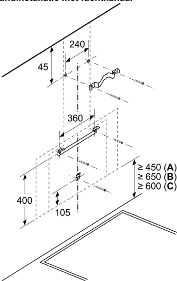
Afmeting in mm Wandinstallatie met luchtkanaal
