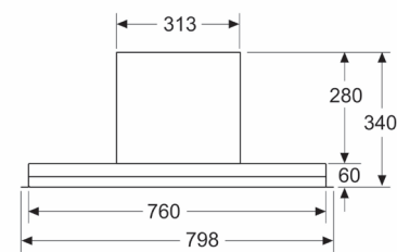
Afmeting in mm Vooraanzicht
